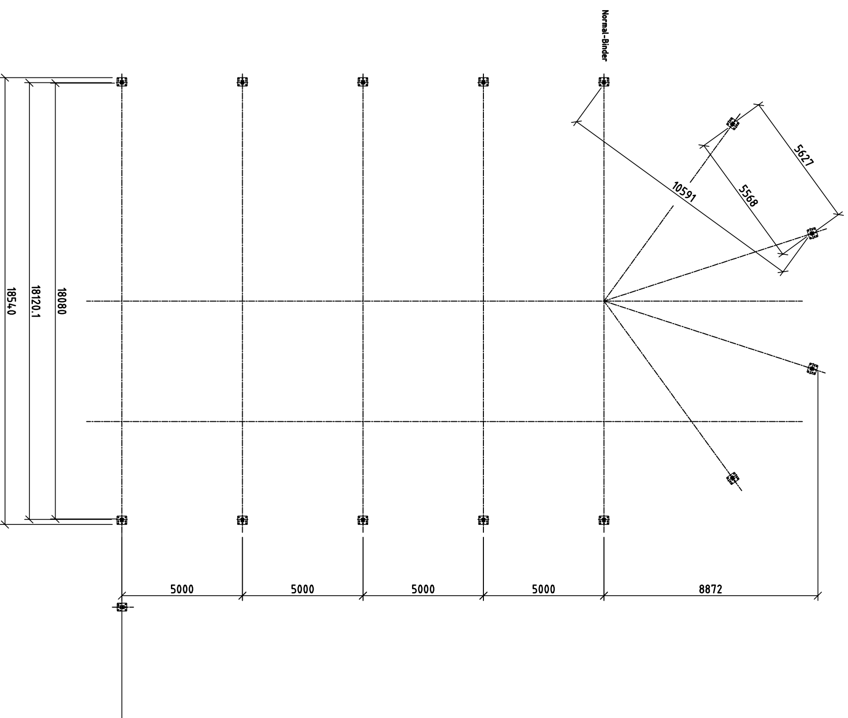
Bodenplattenanordnung Apsis 18,3/...
